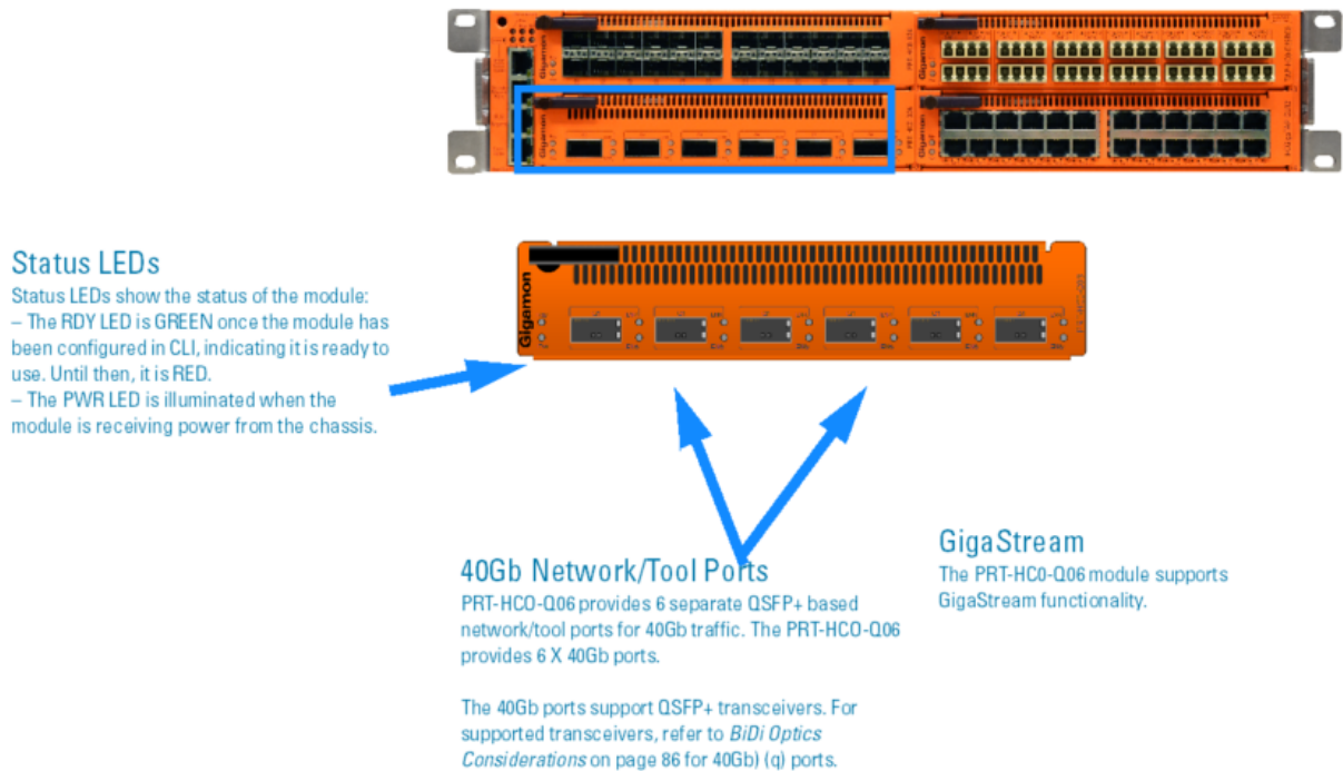
Figure 5 PRT-HC0-Q06 Module
